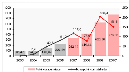
Evolució de la potència eòlica instal·lada a Catalunya 2003-2010 En milions de watts
