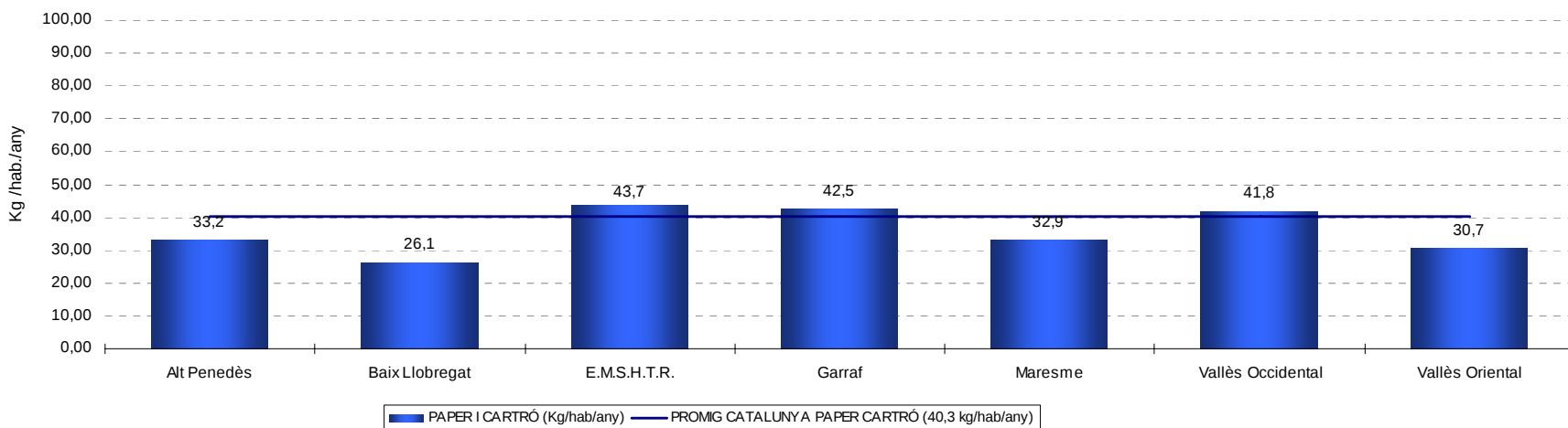
RECOLLIDA SELECTIVA DE PAPER CARTRÓ 2008 (kg/hab/any) PER COMARQUES
