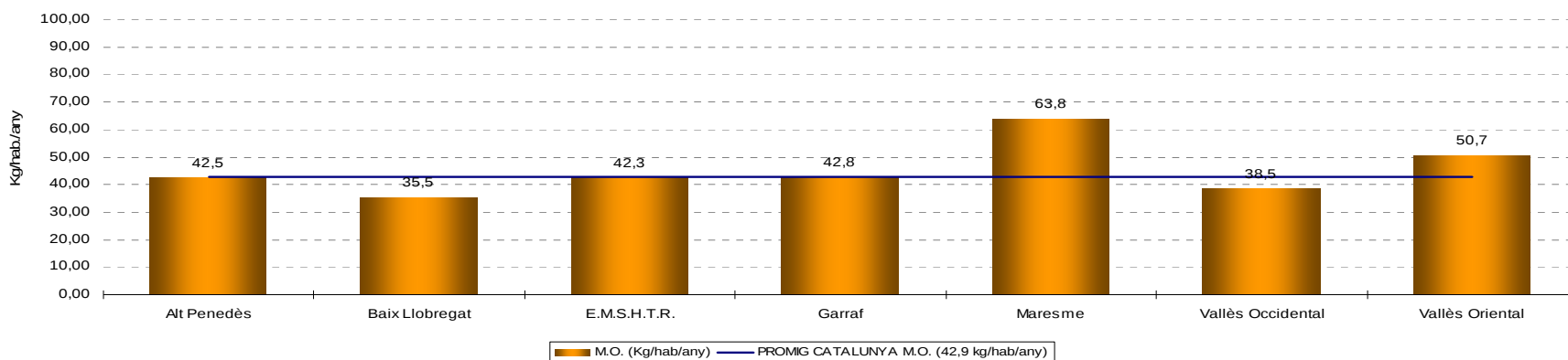
RECOLLIDA SELECTIVA DE FRACCIÓ ORGÀNICA 2008 (kg/hab/any) PER COMARQUES
