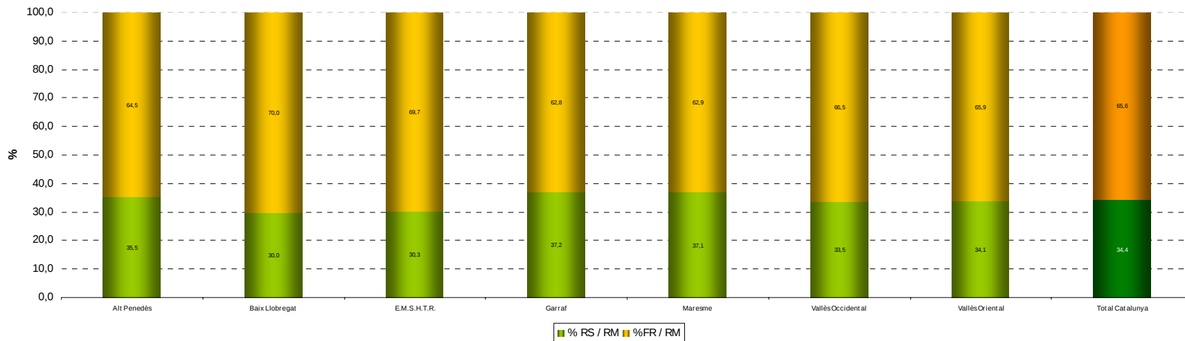
RELACIÓ ENTRE RECOLLIDA SELECTIVA I FRACCIÓ RESTA (%) PER COMARQUES. DADES DE 2008
