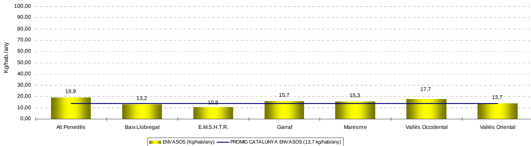
RECOLLIDA SELECTIVA D'ENVASOS 2008 (kg/hab./any) PER COMARQUES
