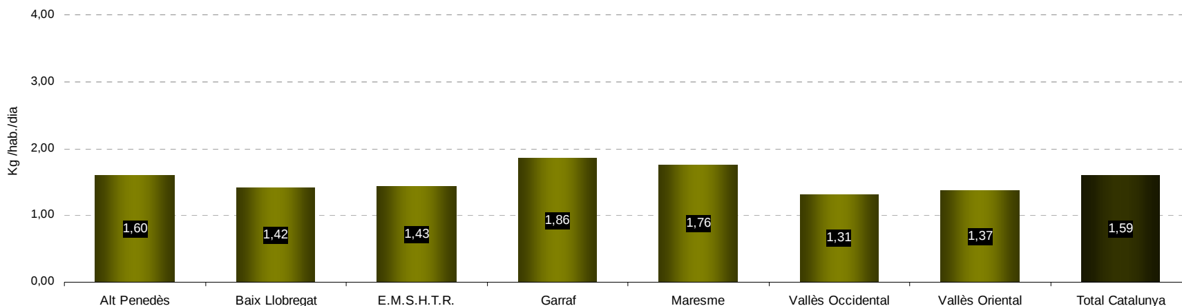
TOTAL GENERACIÓ DE RESIDUS MUNICIPALS (kg/hab/DIA) PER COMARQUES. DADES DE 2008
