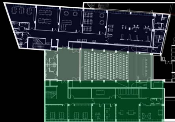
PLANTA SOTERRANI
