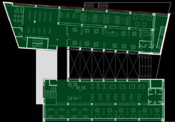
PLANTA ALTELL
