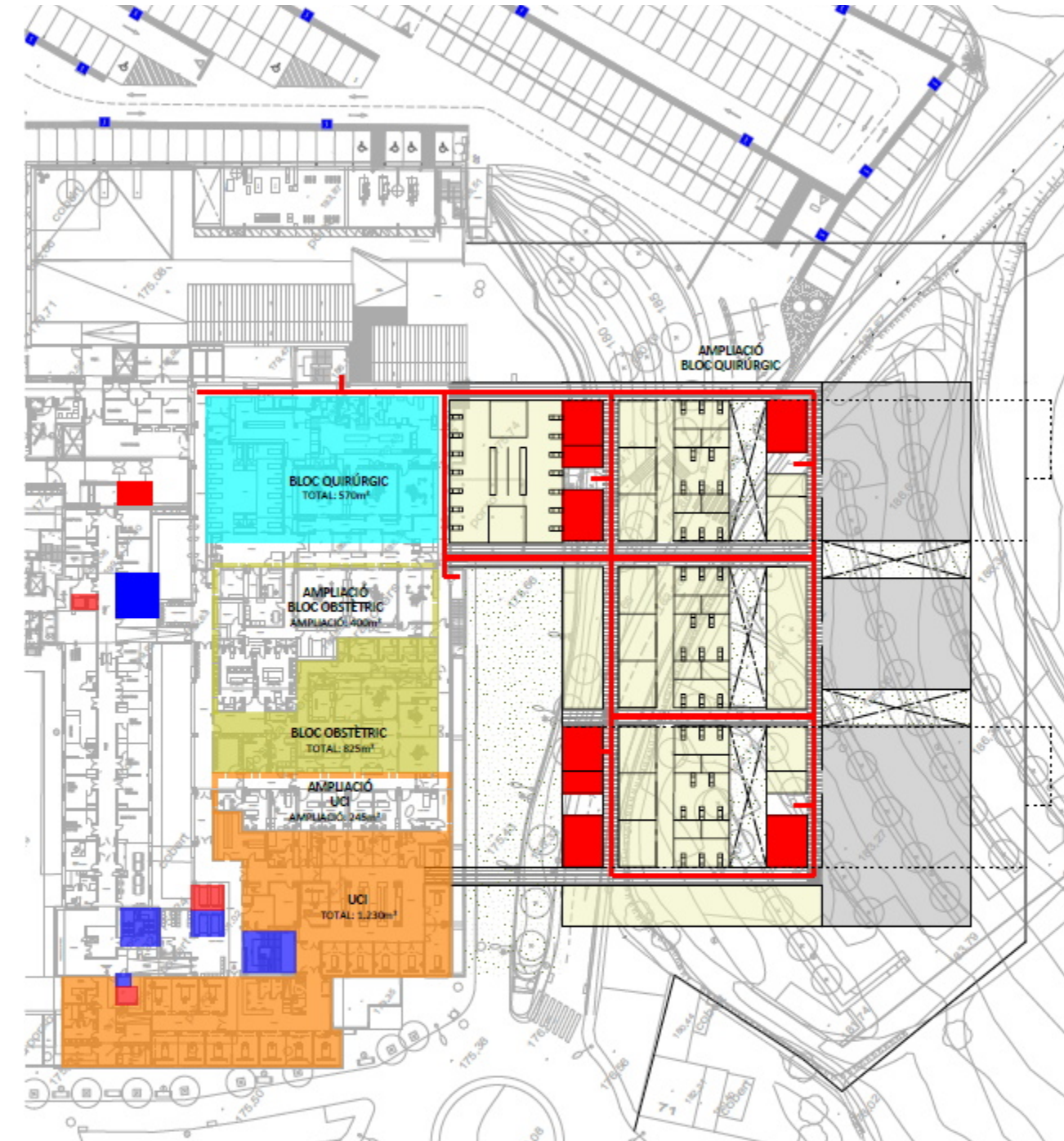
PLANTA PRIMERA – FASE 1
