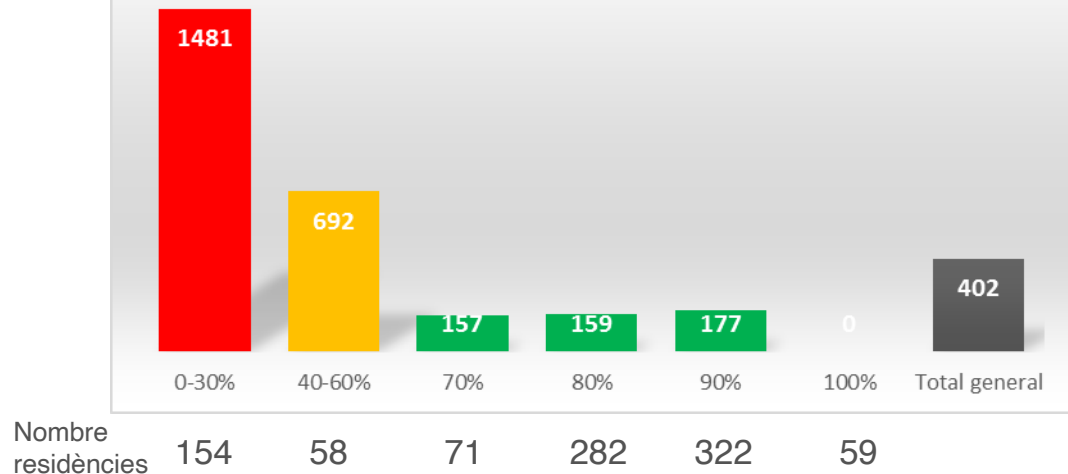
Taxa casos 7 dies /100.000 en relació al % de cobertura amb 2 dosi
