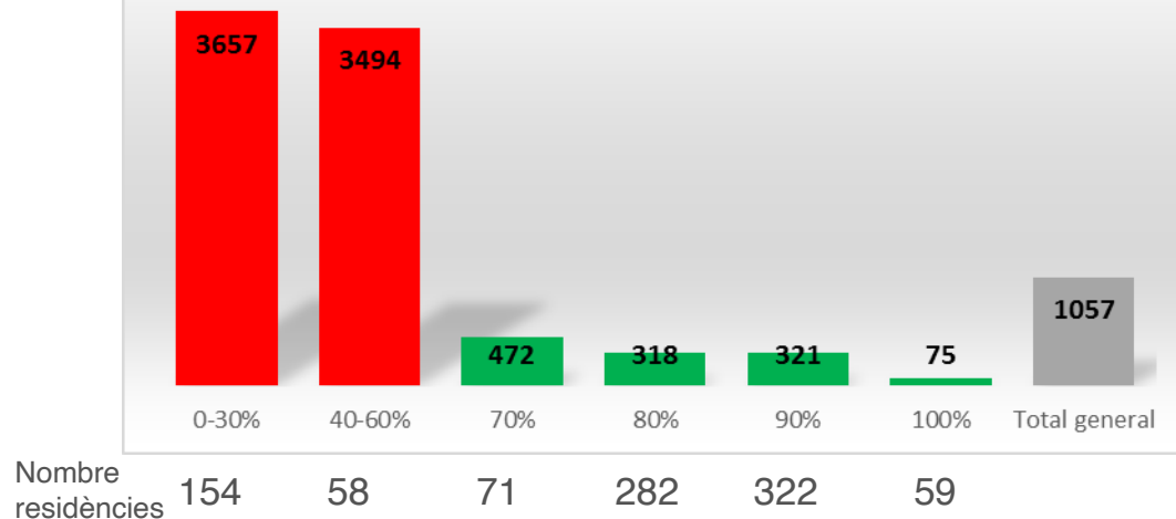
Taxa casos actius /100.000 en relació al % de cobertura amb 2 dosi
