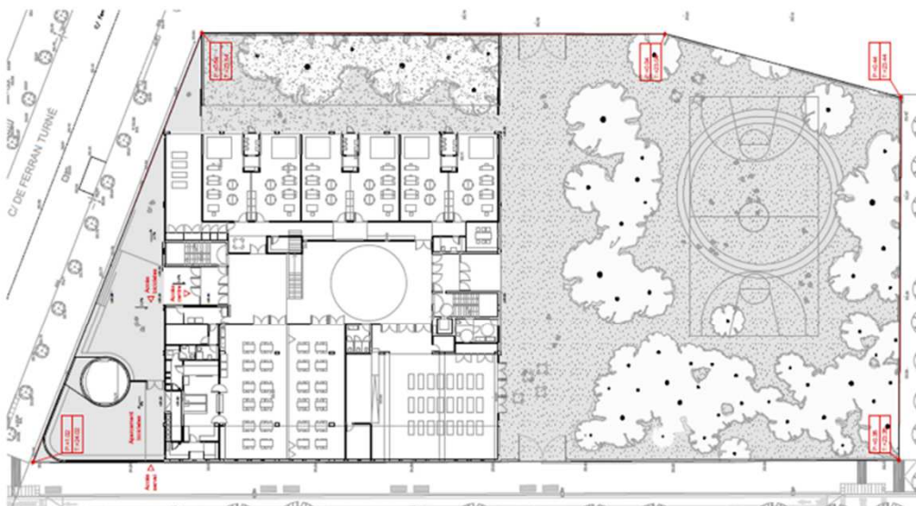
Planta general d'accés
