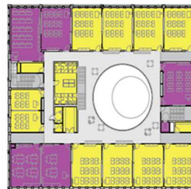
Planta 3
