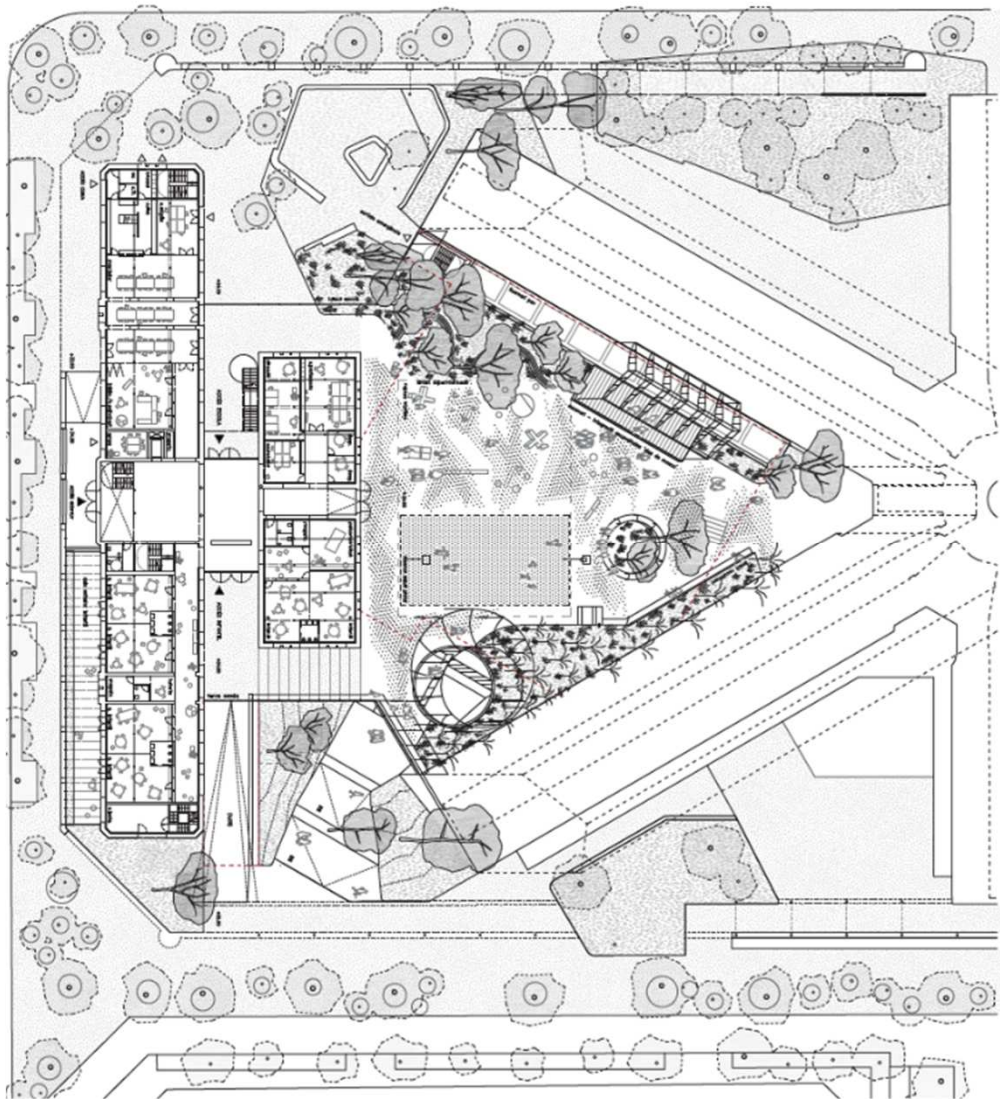
Planta Baixa general
