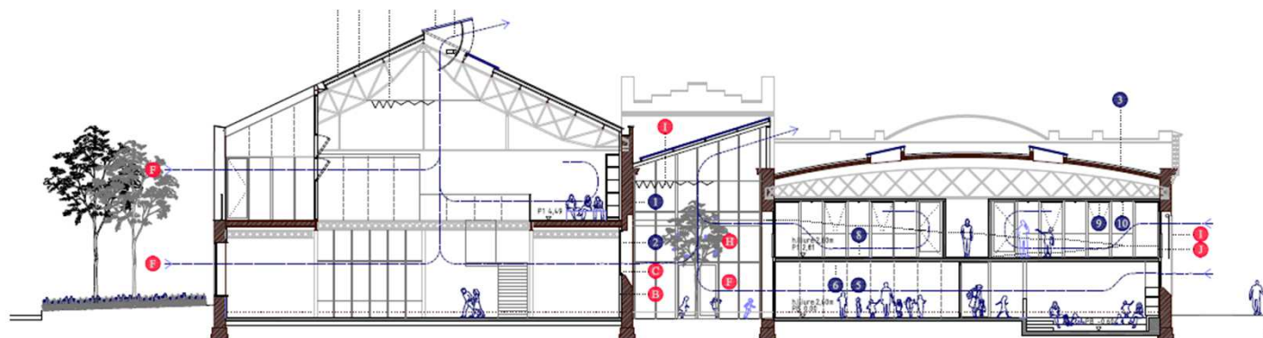
Secció Longitudinal
