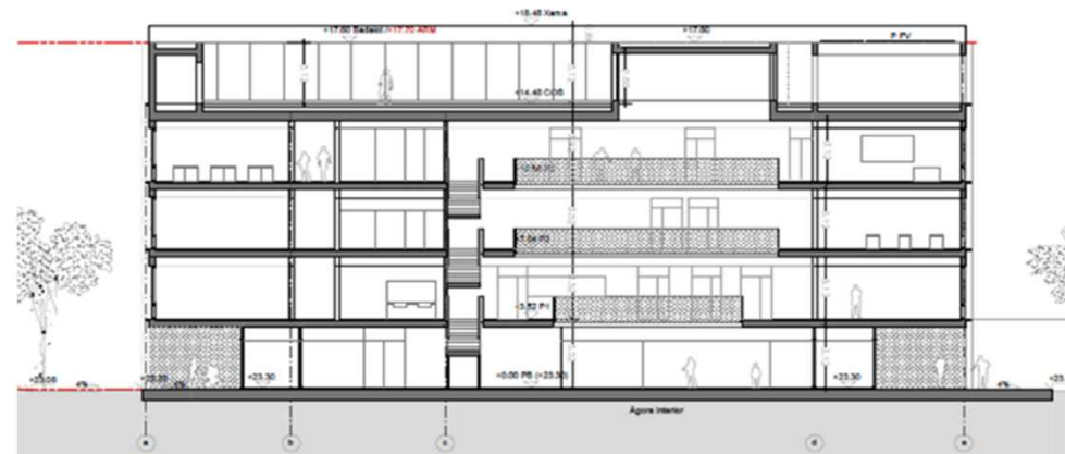
Secció Longitudinal
